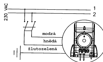
elektrické zapojení
