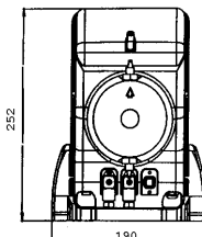
rozměry
