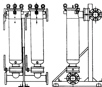
ZDVOJENÝ FILTR s uzavíracími klapkami
